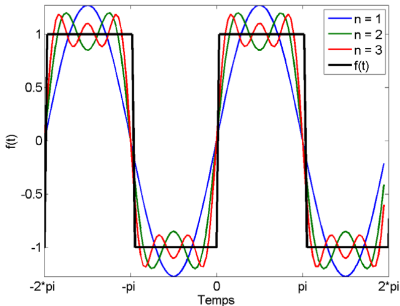
Figure. Phénomène de Gibbs (overshoot, ou ringing).
